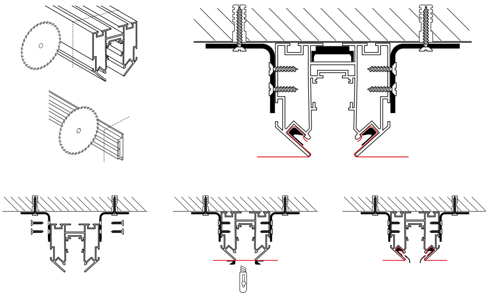
Рис. 2. Установка трека и монтаж натяжного потолка
